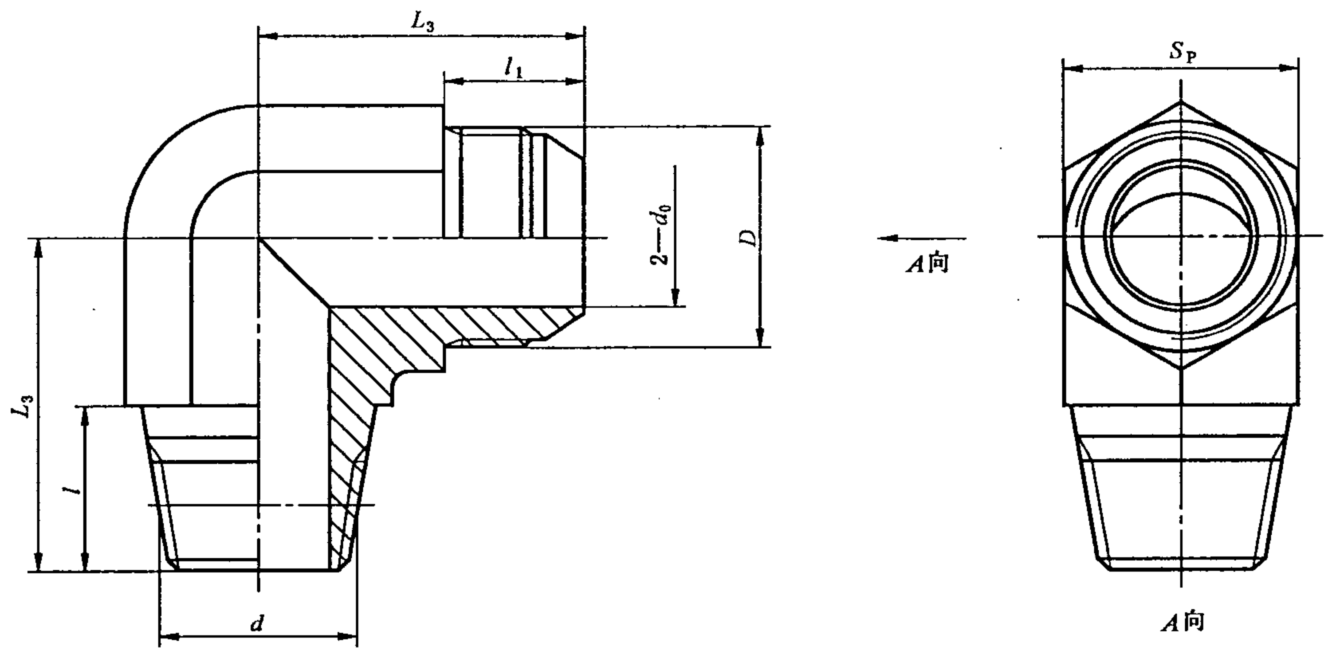
图 4 扩口式锥螺纹弯通接头体
