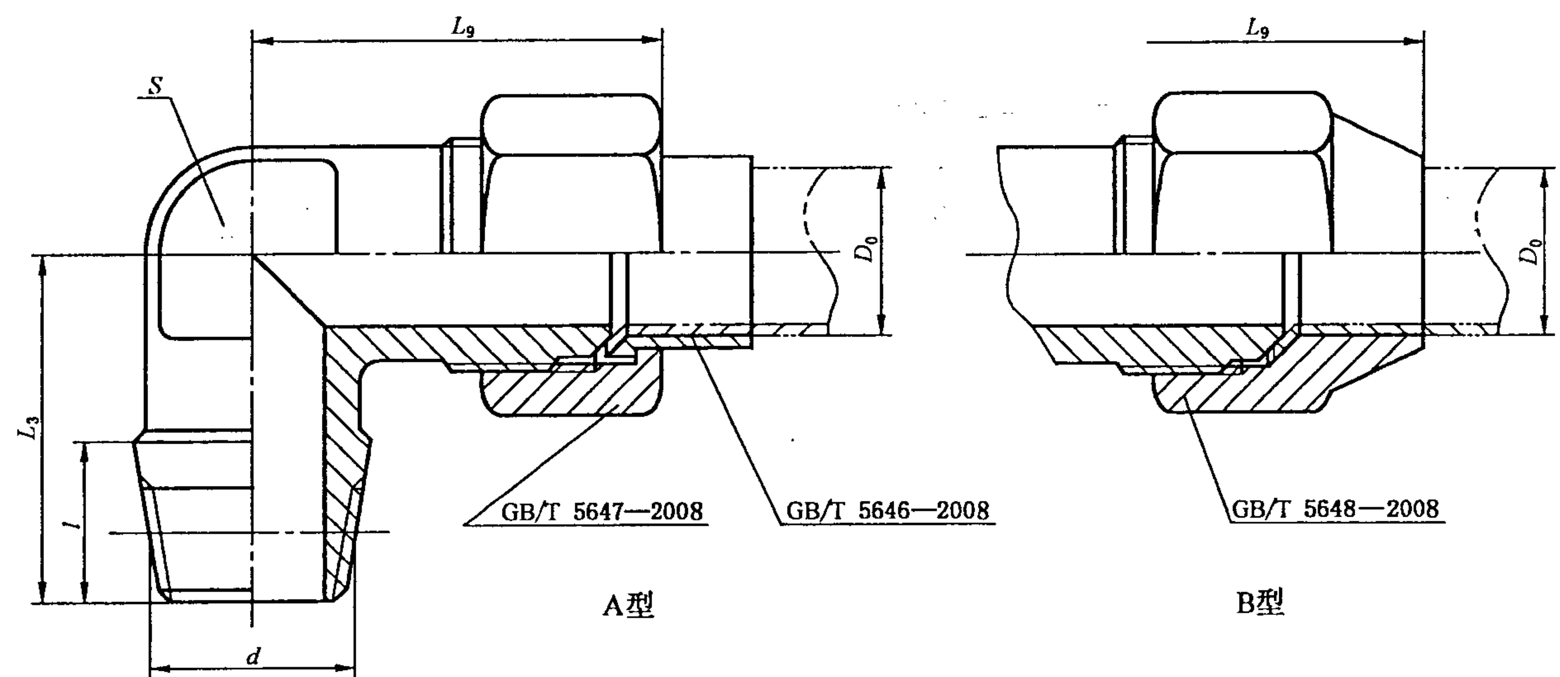
图 1 扩口式锥螺纹弯通管接头
